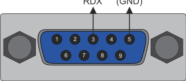
Diagrama de conexión Conexion a Visor Remoto
