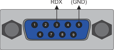
Diagrama de conexión Conexion a Visor Remoto
